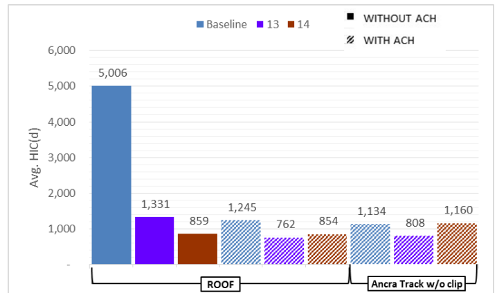
Figure 10: Trim Buck HIC(d)
