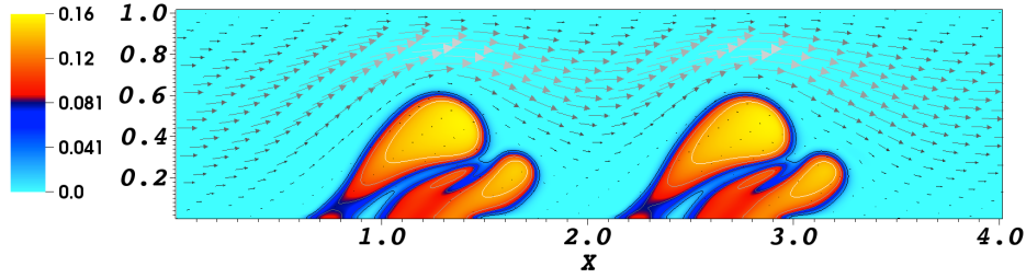
(d) 2D slice of \phi_n at z = 0.35
