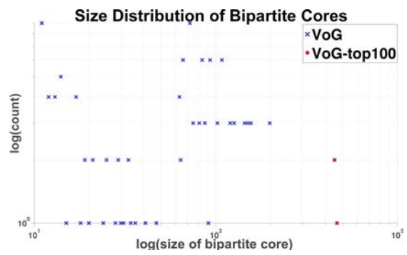
(d) Bipartite cores.
