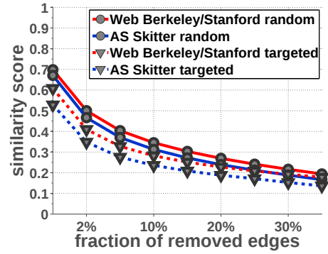
(d) Web Berkeley/Stanford and AS Skitter
