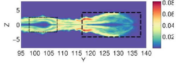
(d) Roughness, t = 55.0
