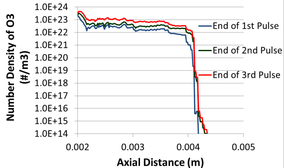
O 3 density
