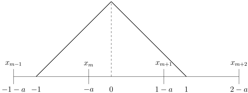
FIGURE 1. S(x) = 1 - |x|, |x| < 1, S(x) = 0, |x| \geq 1
