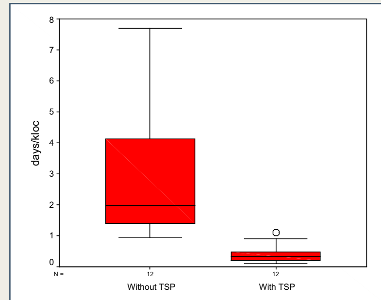
Test Time per KLOC
