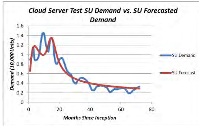
Figure 27. SU Forecaset—Cloud Server Model.
