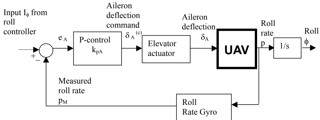
Fig. 2.4 Roll damper
