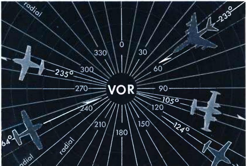
FIGURE 125 VOR radials
