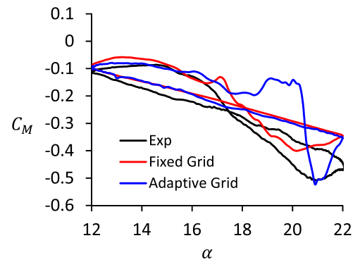
(d) r/R = 0.99
