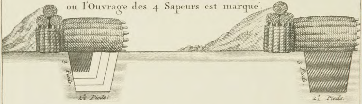
Gabion farci.
