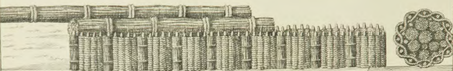
Veue du dedans d'une Sape sur sa longueur.
