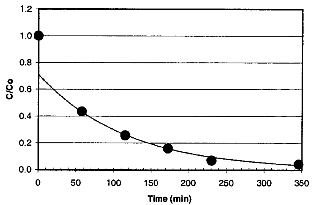
Moffett - TCE Profile 6 317 PVs
