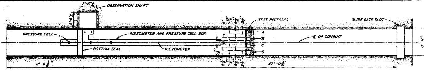
SECTION A-A
