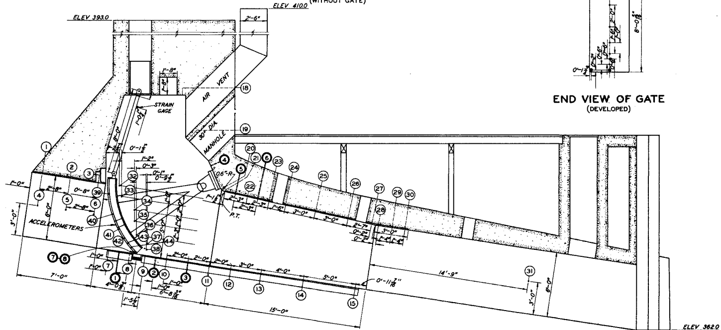
SECTION A-A
