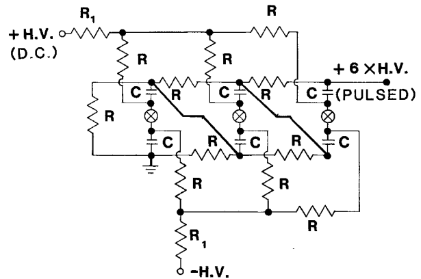
H.V. MARX GENERATOR
