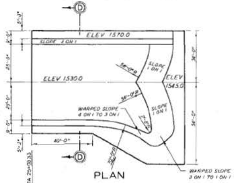
TYPE DI DESIGN
