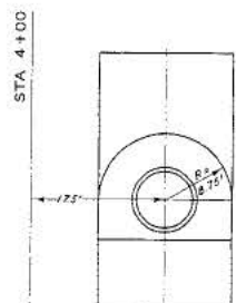
SECTION D-D
