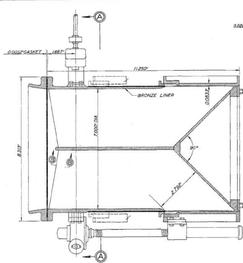
ELEVATION
