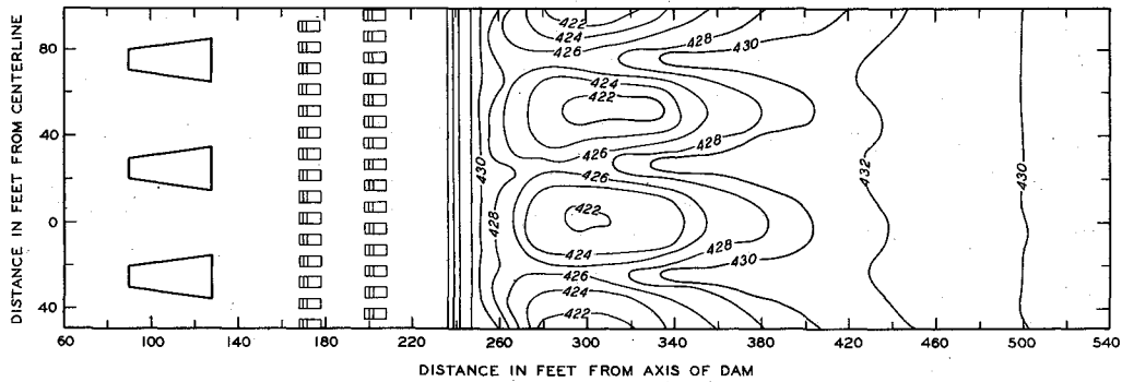
SCOUR PATTERN
