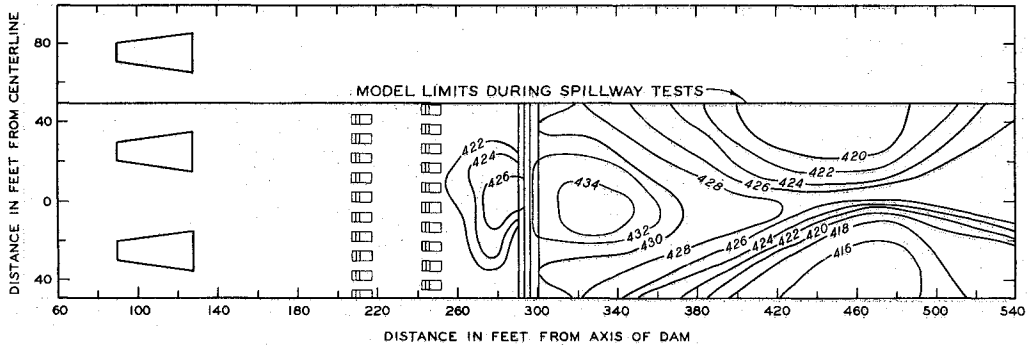
SCOUR PATTERN
