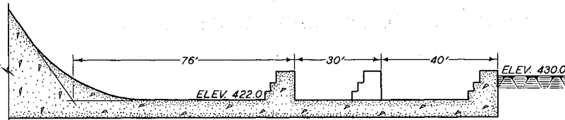
TYPE 2 APRON
