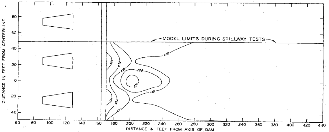
SCOUR PATTERN
