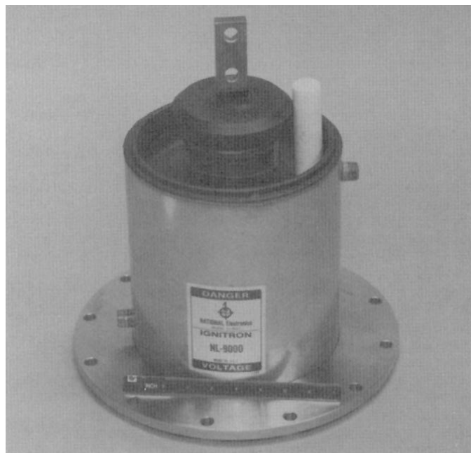
Fig 3-NL-9000 Ignitron.
