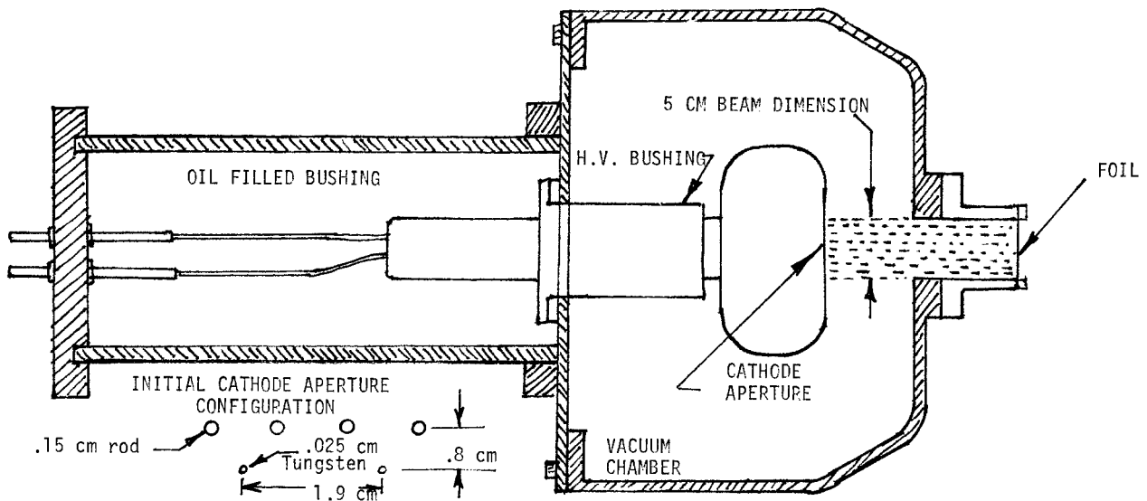
Fig. 2 E-Gun Configuration
