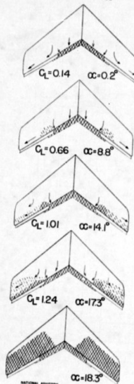
(d) Upper-surface flaps and extended split flaps on.
