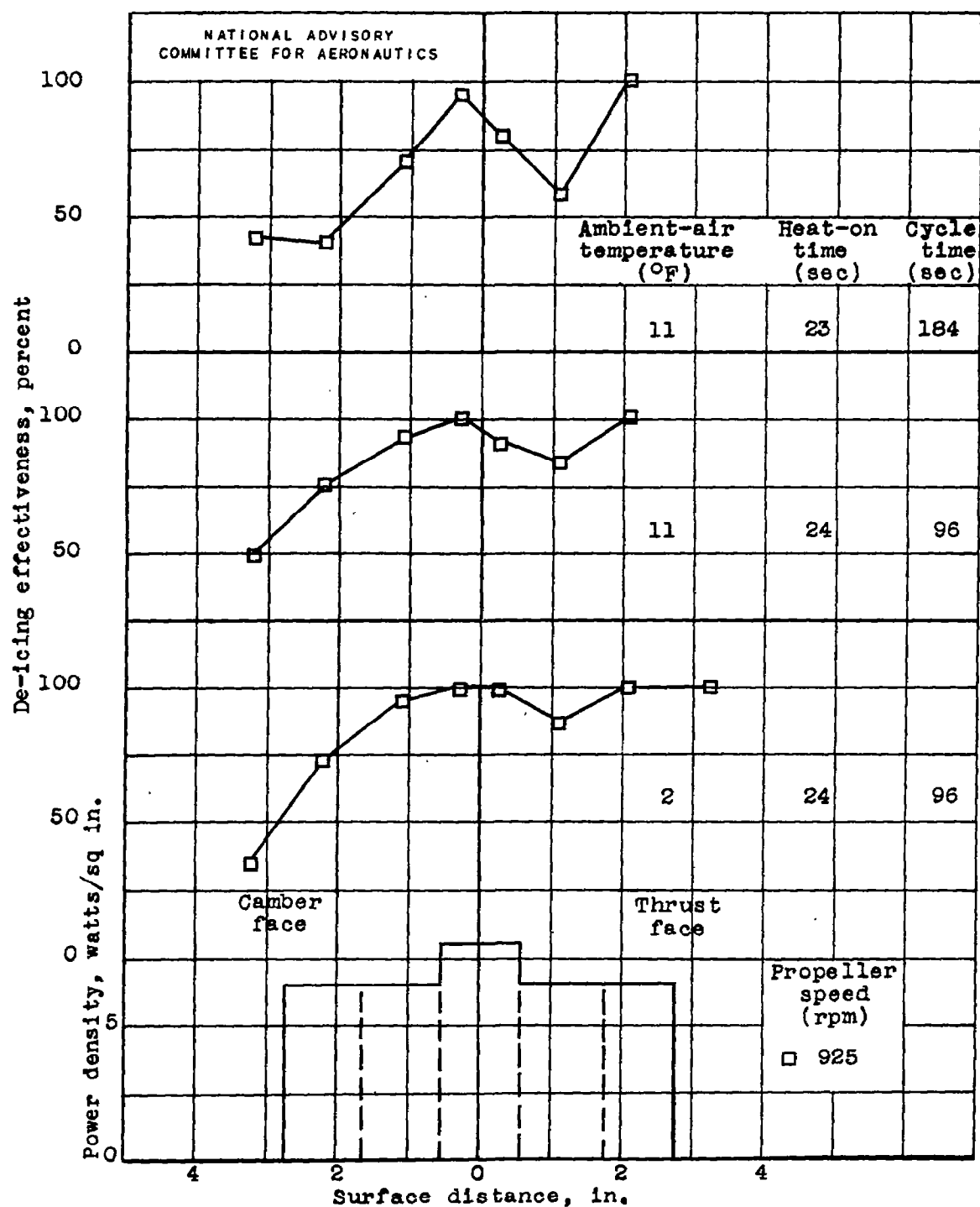
(d) Heating pattern 4.
