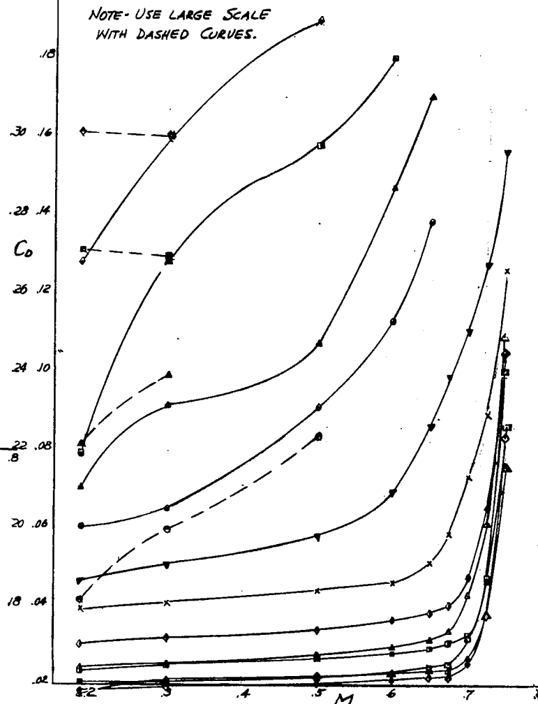
(d) Variation of C_L and C_D with Mach number.
