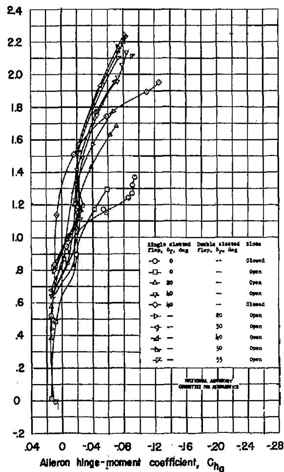
(d) Aileron hinge-moment characteristics.
