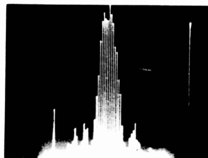
20 MC/SEC 0.10 \mu SEC R. F. SPECTRUM
