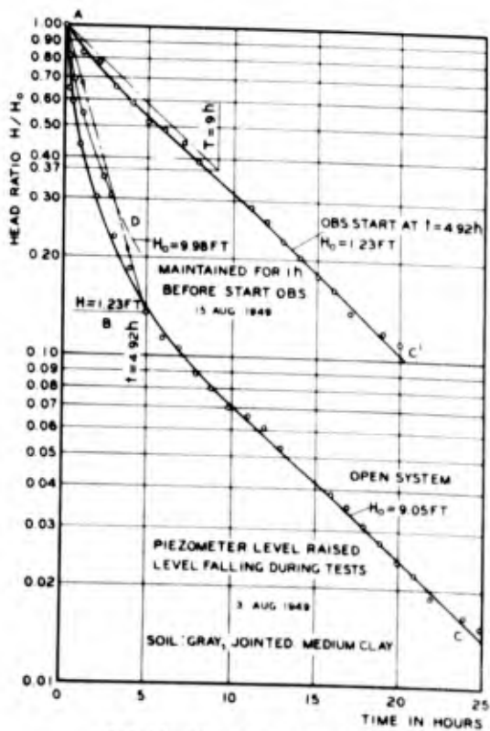
CASAGRANDE TYPE PIEZOMETER FIG. 15-B
