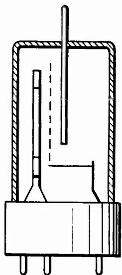
Figure 16. Vibrotron.
