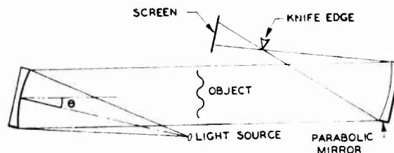
Figure 26. Schlieren apparatus.
