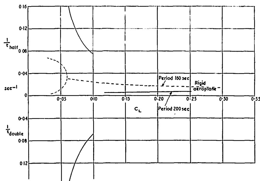
FIG. 9a. 'Phugoid' mass distribution A.
