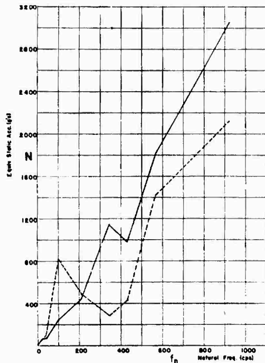
Fig. 8 - 3-foot back blow
