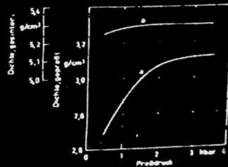
Bild 2 Dichte von gepreßten (a) und von gesinterten (b) Ferritteilen
