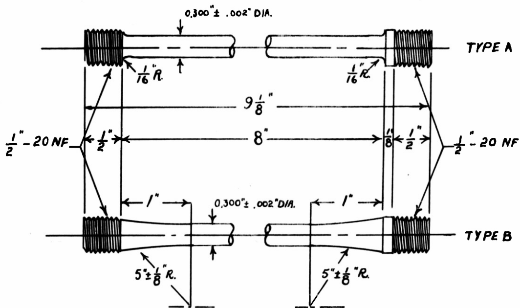
Fig. 3. Tensile specimens.
