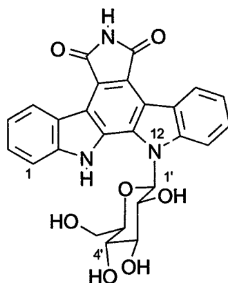
Deschlororebeccamycin-aglycone
