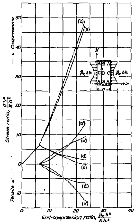
(a) \sigma_x b^2/Eh^2 (A) (b) \sigma_x b^2/Eh^2 (B) (c) \sigma_x b^2/Eh^2 (C) (d) \sigma_x b^2/Eh^2 (D) (a') \sigma_y b^2/Eh^2 (A) (b') \sigma_y b^2/Eh^2 (B) (c') \sigma_y b^2/Eh^2 (C) (d') \sigma_y b^2/Eh^2 (D)
