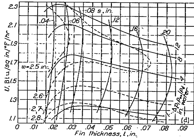
(d) Fin weight M , 0.3334 pound per square inch wall area.
