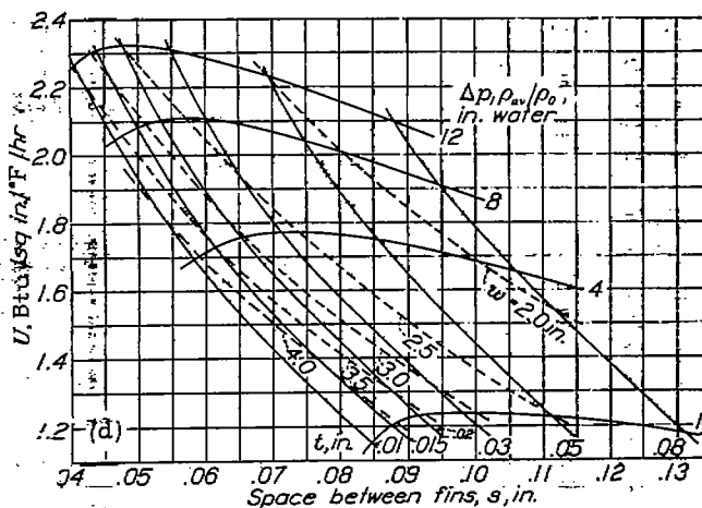
(d) Fin weight M , 0.3384 pound per square inch wall area.
