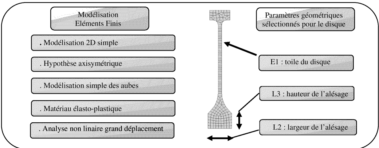
Figure 6 – paramétrage et maillage du disque
