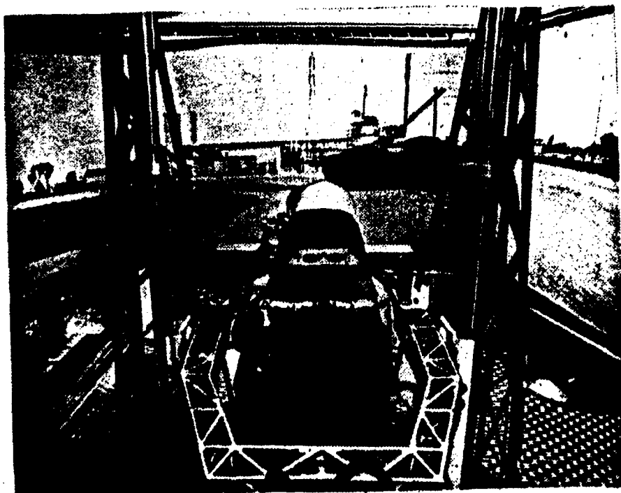
FIG. 19. DISPLAY SYSTEM
